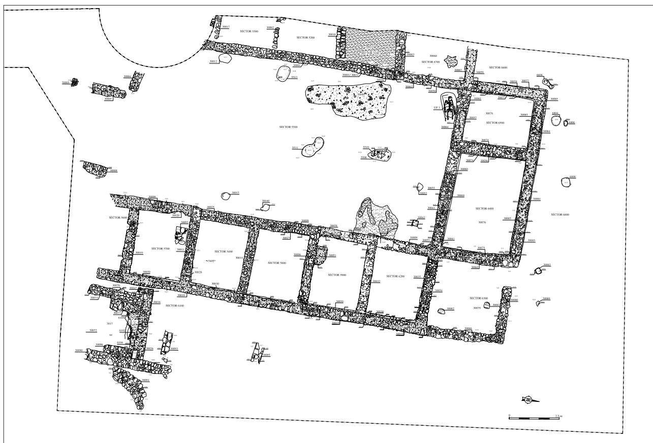
FIGURA 3. Planta general de l'edifici septentrional localitzat dins de l'àrea 3000. Planimetria a càrrec de Codex, Arqueologia i Patrimoni.
