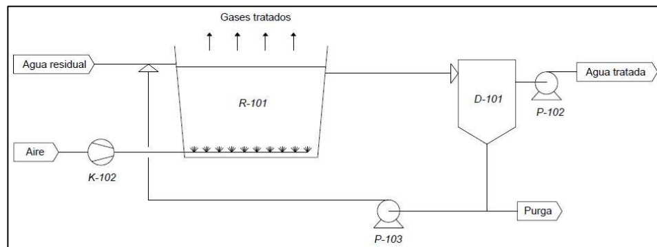
Figura 2.5. Esquema reactor biológico.
