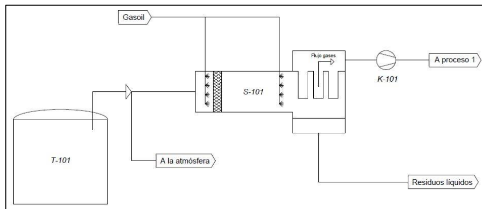
Figura 2.1. Esquema proceso 0.
