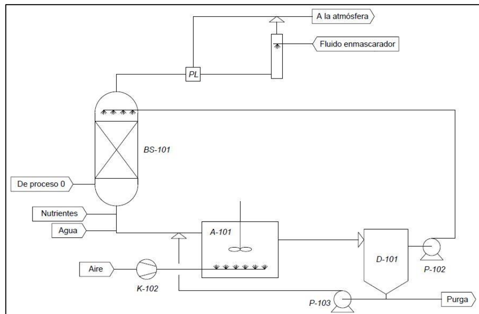
Figura 2.3. Esquema bioscrubber .
