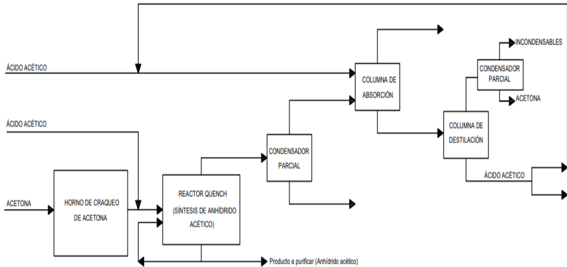
Figura 3.1. Diagrama de bloques del proceso.
