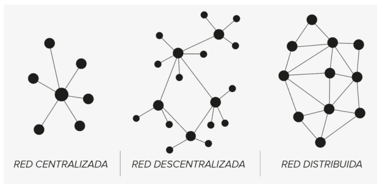
Ilustración 2. Tipos de red
