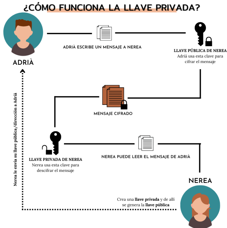
Ilustración 5. Funcionamiento de la llave pública y la llave privada en una transacción
