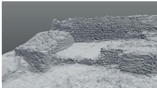
FIGURA 1. Detalle del modelado 3D a partir de vuelos con dron sobre la torre número 5. Se aprecia la forma irregular de cimentar la estructura.
