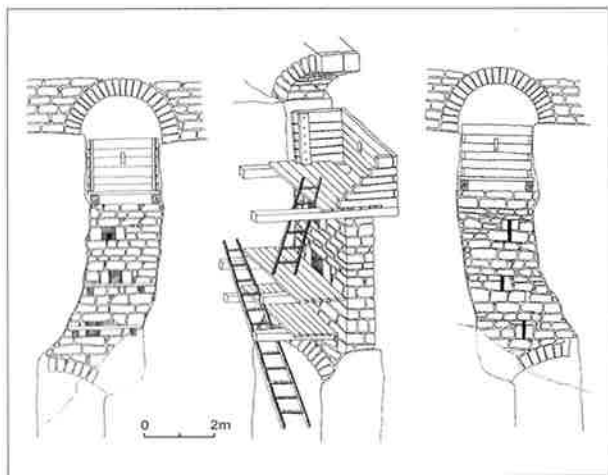
Figura 4: reconstrucció idealitzada de l'estructura de fusta interna i del sistema defensiu de l'accés. (J. Zaragoza).
