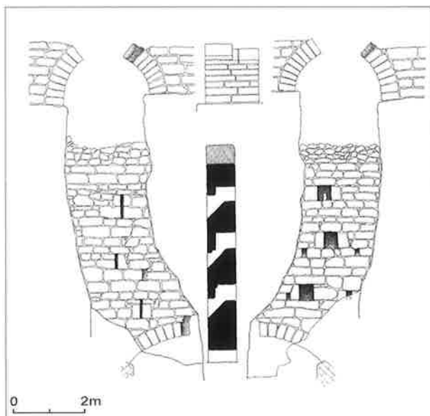
Figura 3: alçats i secció del pany de muralla oriental on hi ha l'accés. (J. Zaragoza).
