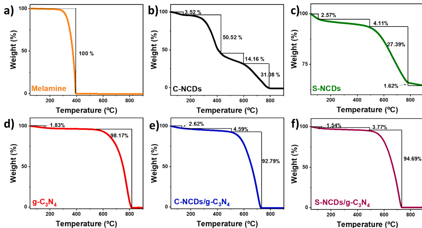
Fig. 2. TGA: a) melamine, b) C-NCD, c) S-NCD, d) g-C 3 N 4 , e) C-NCD/g-C 3 N 4 and f) S-NCD/g-C 3 N 4 .
